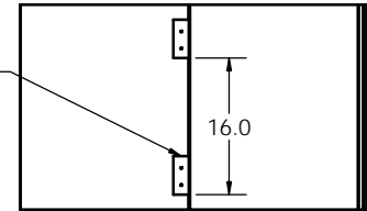
AGRAFFES INTERMITANTES
